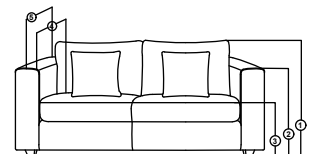
1). TOTAL HEIGHT - 33.75" (85.5cm) 2). ARM REST HEIGHT - 27" (68.5cm) 3). SEAT HEIGHT - 15.75" (40cm) 4). SEAT DEPTH - 22.75" (58cm) 5). TOTAL DEPTH - 36" (91.5cm)
