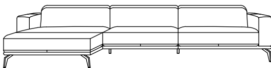
3 STR + RH / LH DAYBED TW - 123" / ISW - 106" TW - 312cm / ISW - 269cm DBTW - 44"(112cm) / DBISW - 35.5"(90cm) DBTD - 71"(180.5cm) / DBSD - 50.5"(128cm)
